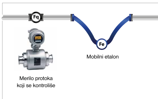
Šema priključenja na cevovod
